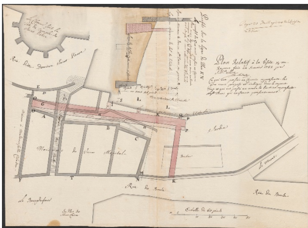
Document numérisé : plan remis par l'Hospice général : projet d'aménagement du petit hôpital, J.-M. Billon, janvier 1752. (AEG Archives hospitalières Ee 9 aaa)
